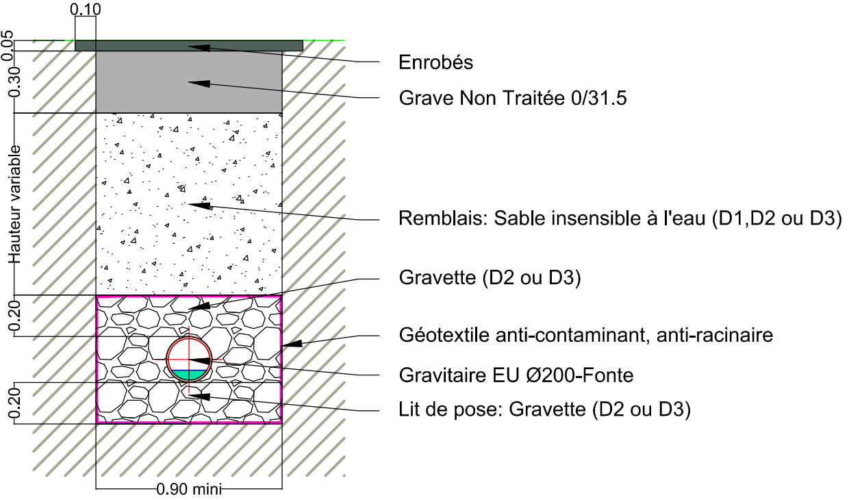
Coupe type de tranchée Routes Communales Présence de nappe
