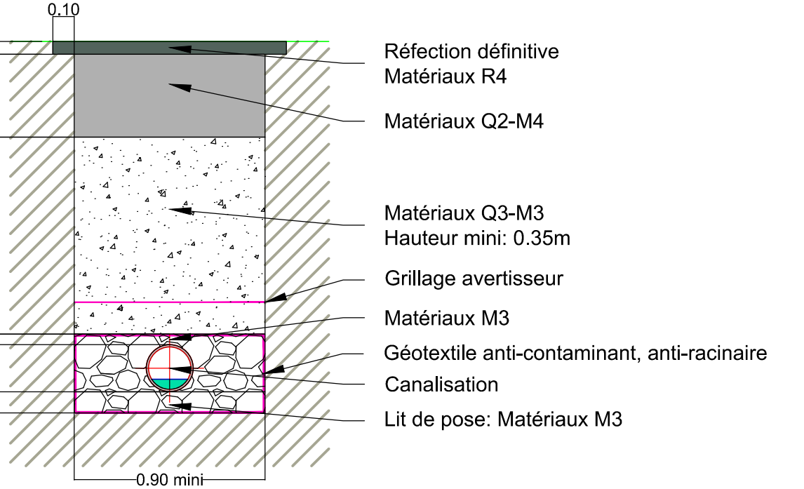
Coupe type de tranchée Route Départementale T1
