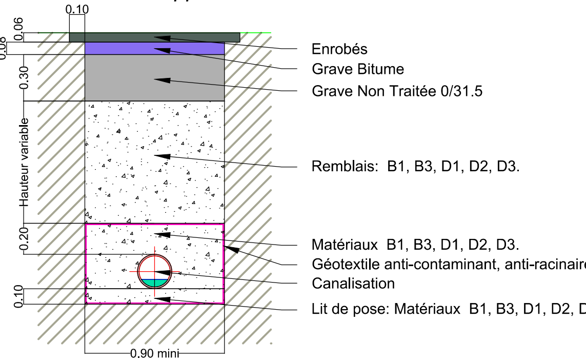
Coupe type de tranchée Route Départementale Hors nappe
