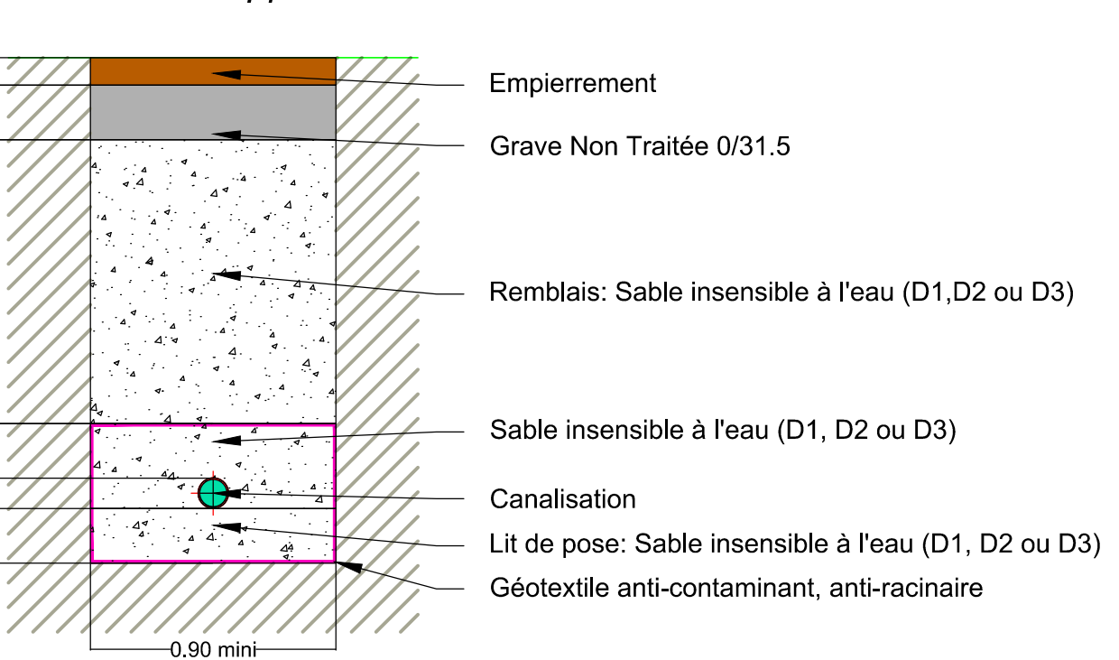
Coupe type de tranchée Chemins empierrés Hors nappe
