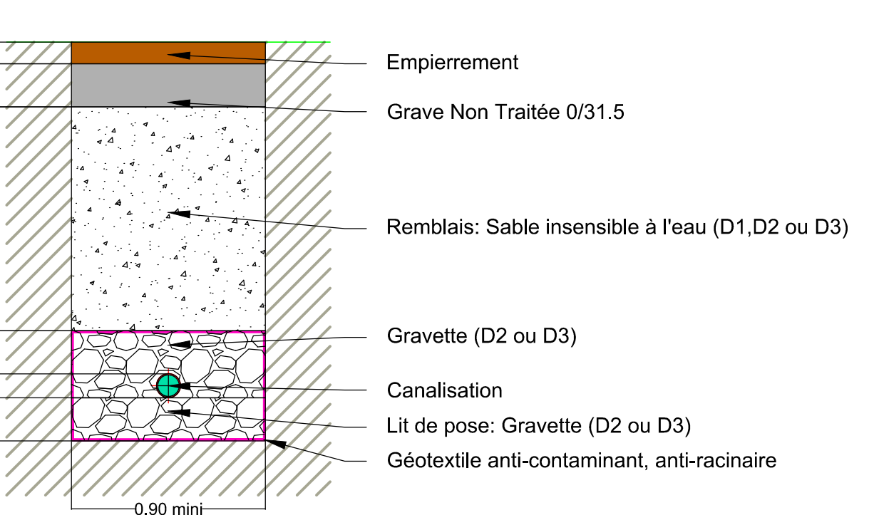
Coupe type de tranchée Chemins empierrés Présence de nappe
