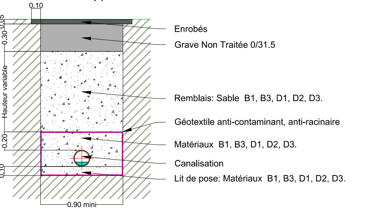
Coupe type de tranchée Branchement Sous-trottoir Hors Nappe
