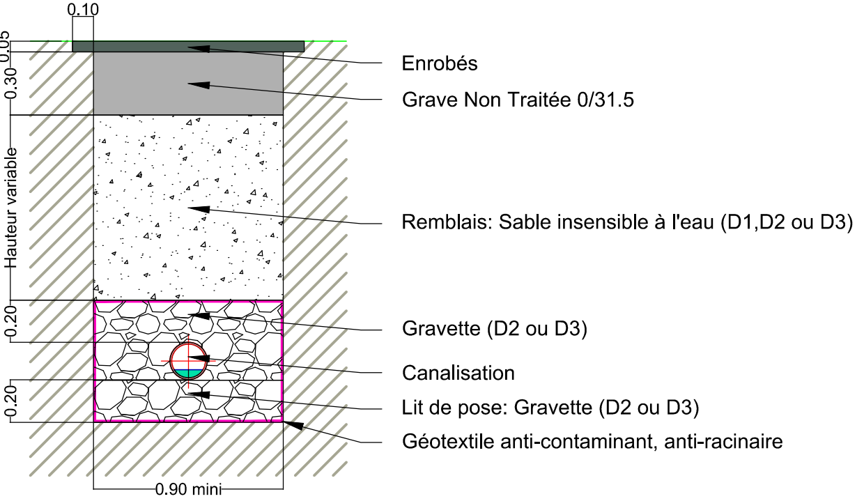
Coupe type de tranchée Branchement Sous trottoir Présence de la nappe
