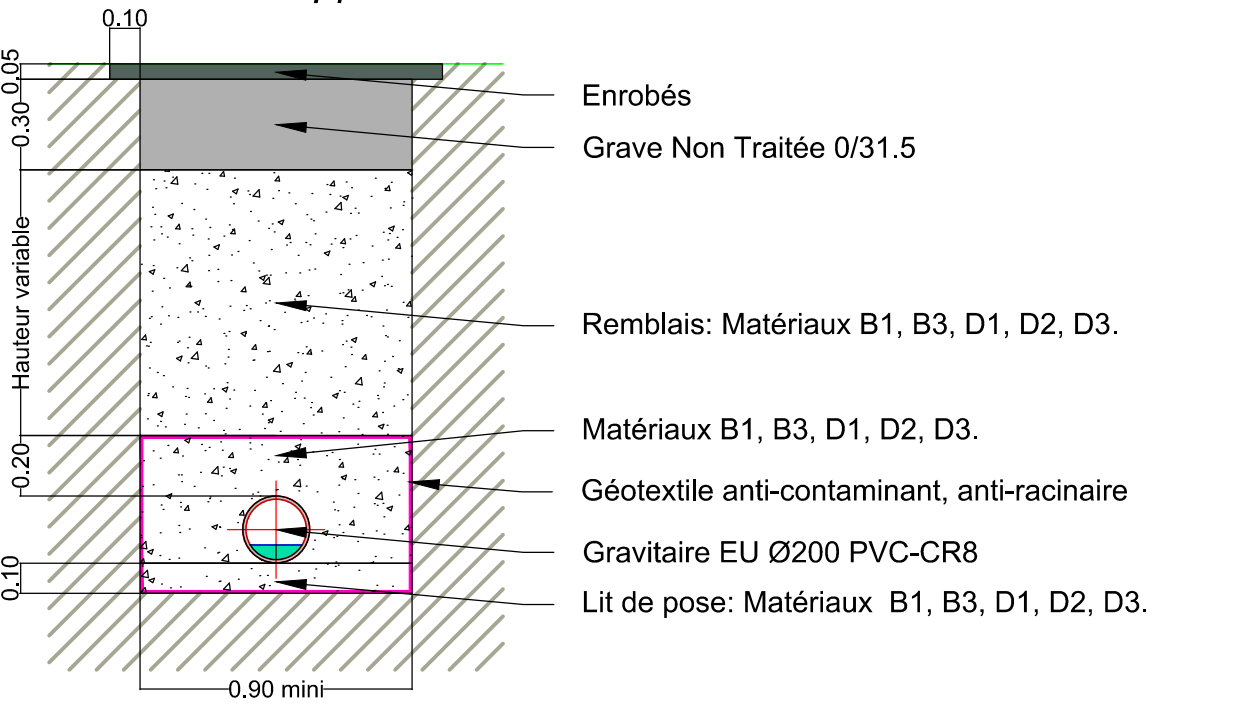
Coupe type de tranchée Chaussée Communale Hors nappe
