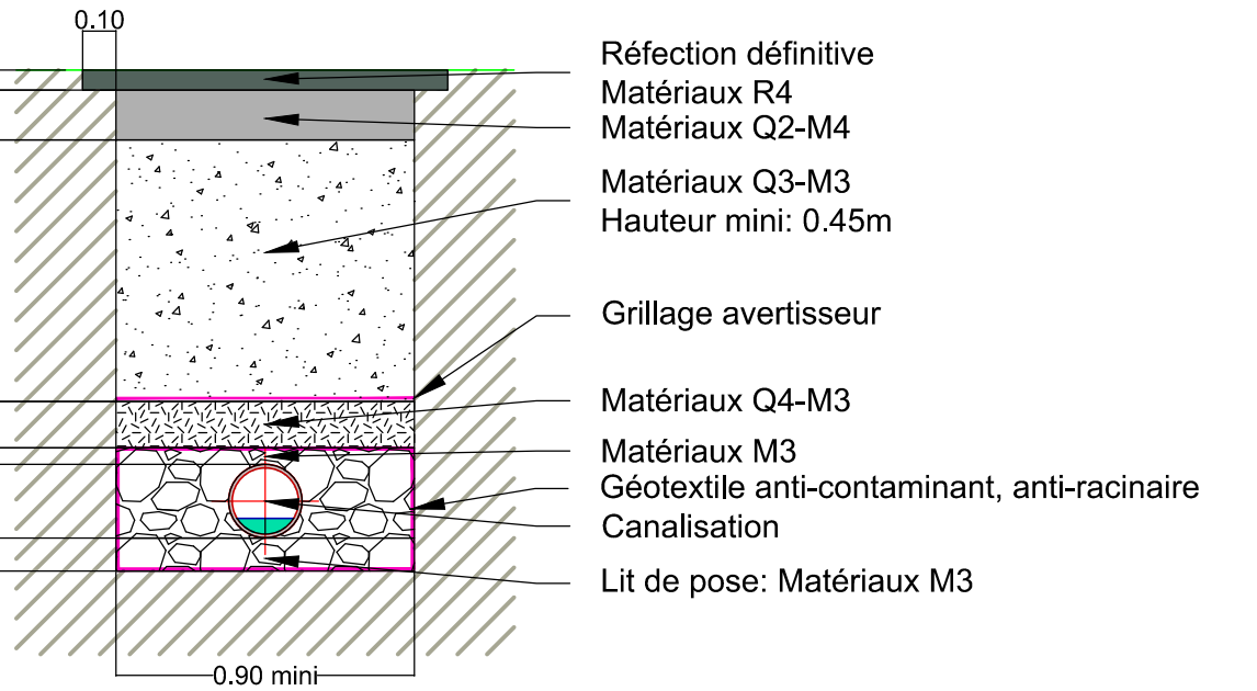
Coupe type de tranchée Route Départementale T3
